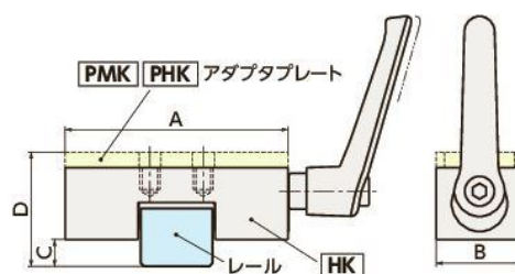
図 2. 選定表記載の寸法図
