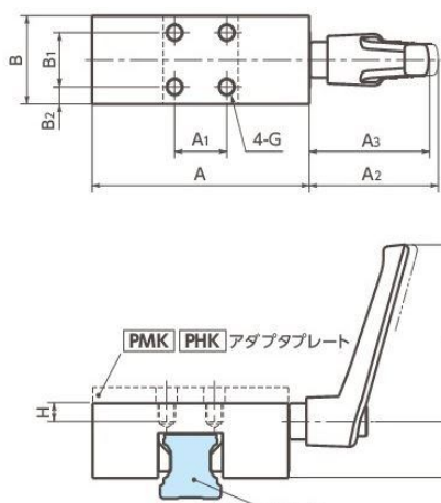
図 1. 寸法表記載の寸法図
