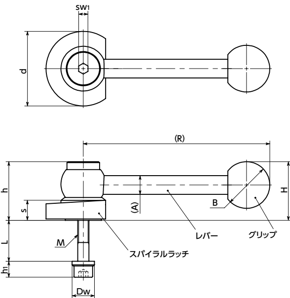
LZY-GVB-A-R 右回転
