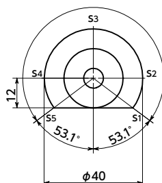
LZY-40-A
