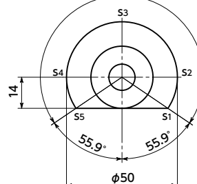
LZY-50-A
