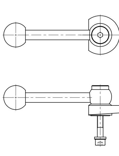
LZYS-GVB-B-L 左回転
