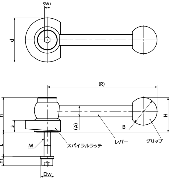
LZYS-GVB-B-R 右回転
