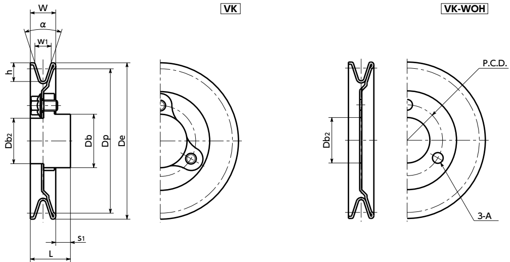
VK ハブつき 単位: mm
